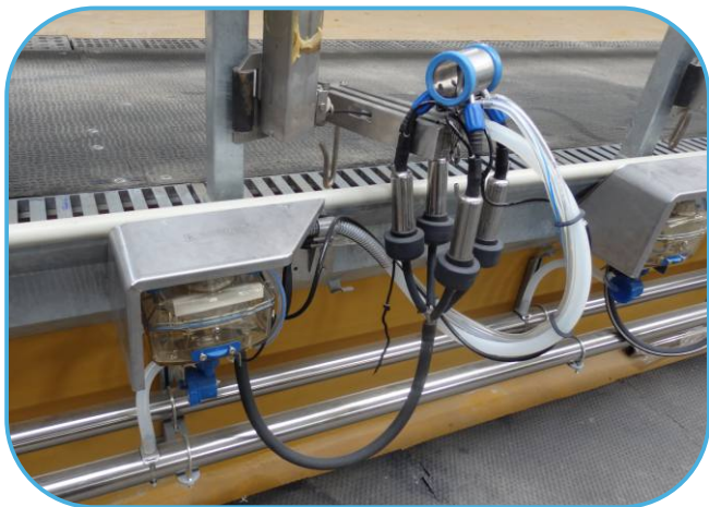
dojící stroj s polohovacím ramenem a měřič nádoje
