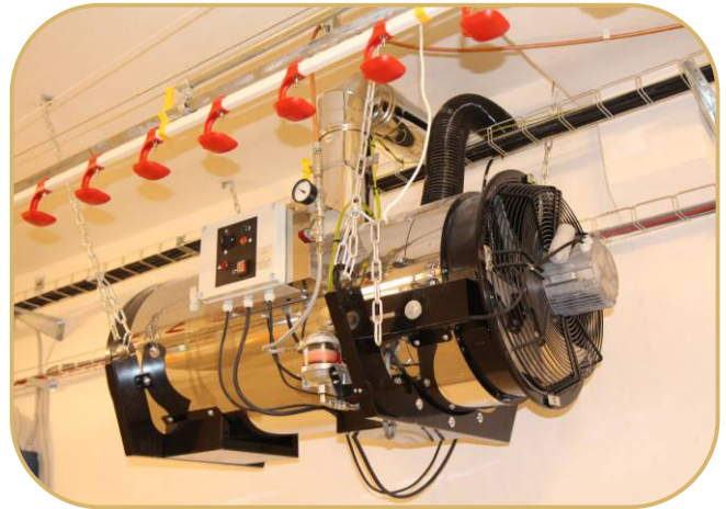
topidlo BH 50 na LTO, s odvodem spalin a přívodem vzuchu
