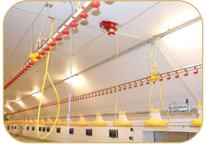
linky krmení, napájení a vysokotlaké chlazení
