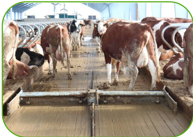
řetězová skládací shrnovací lopata - systém DELTA
