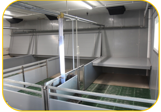
uspořádání kotců v dochovu selat
